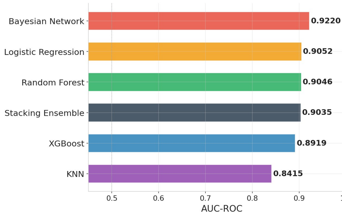
AUC-ROC Comparison
